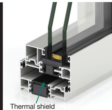
Thermal shield
